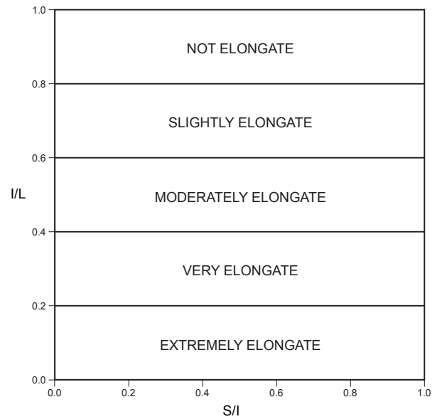
Zingg (1935) diagrams
