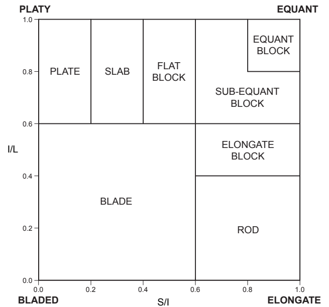
Zingg (1935) diagrams
